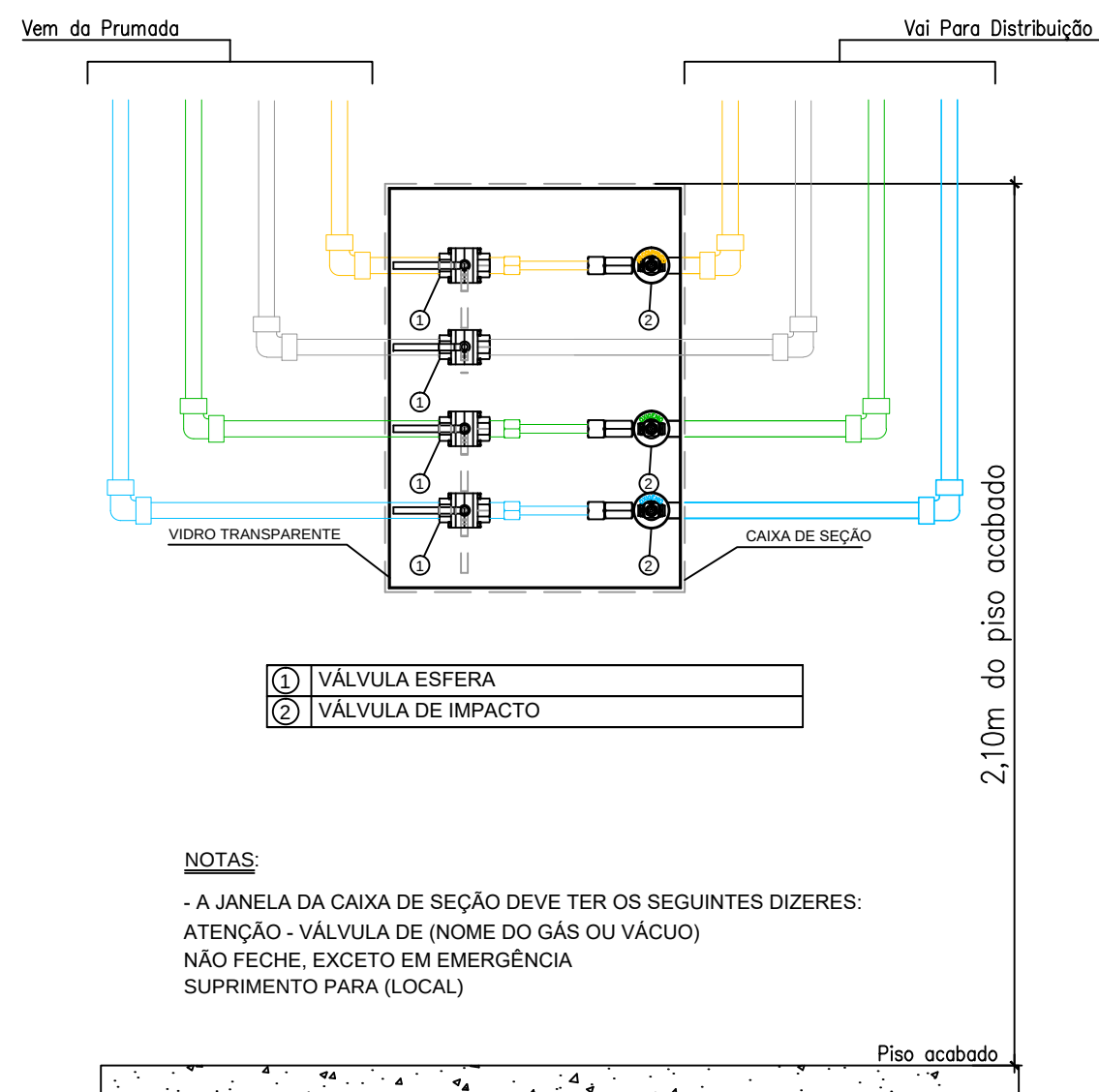
DETALHE 2 – CAIXA DE SEÇÃO SEM ESCALA
