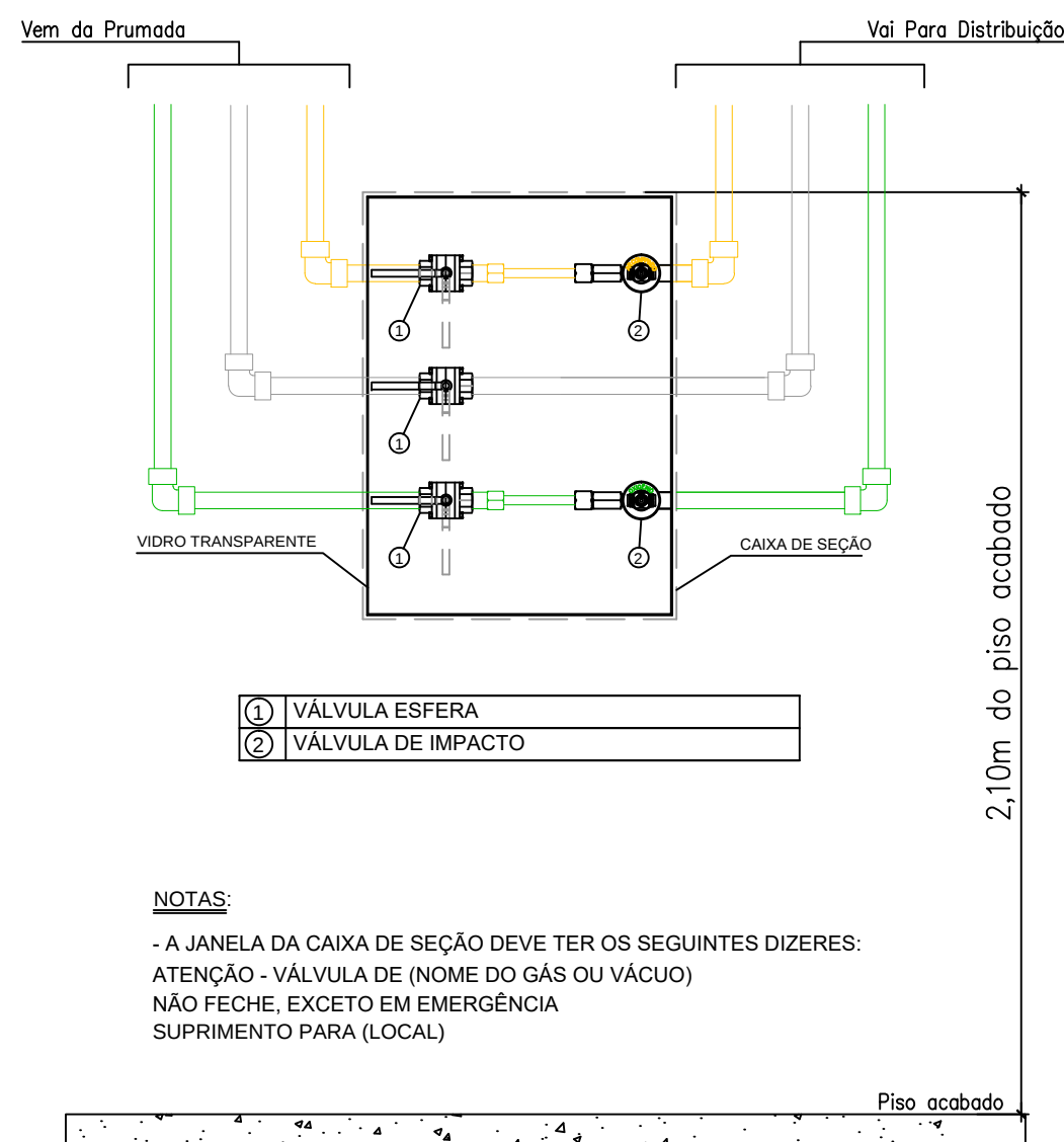
DETALHE 1 – CAIXA DE SEÇÃO SEM ESCALA
