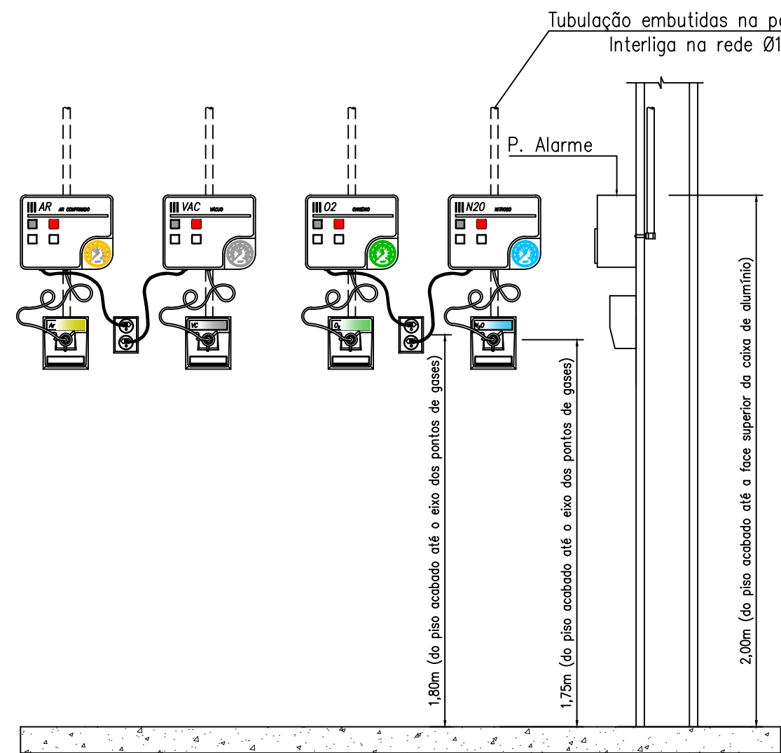
DETALHE 5 – PAINEL DE ALARME SEM ESCALA
