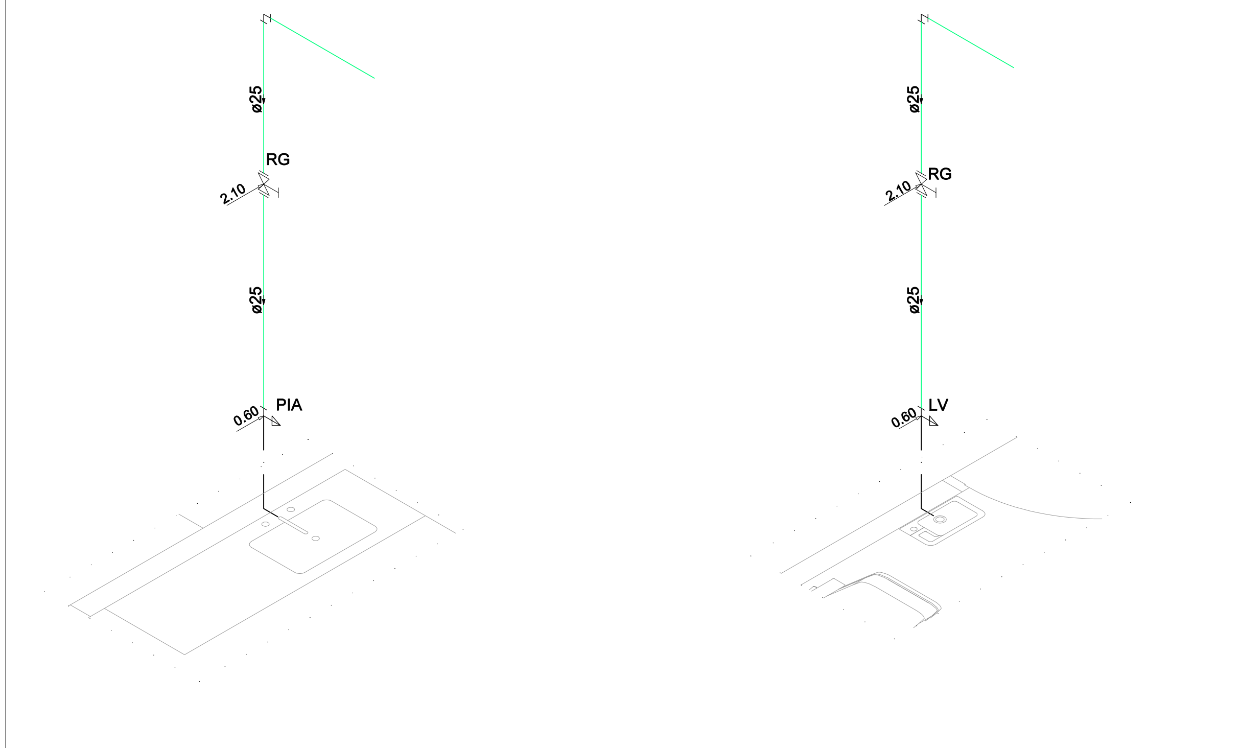
DETALHE ISOMÉTRICOS SANTA CASA FASE 3 ESCALA 1:50
