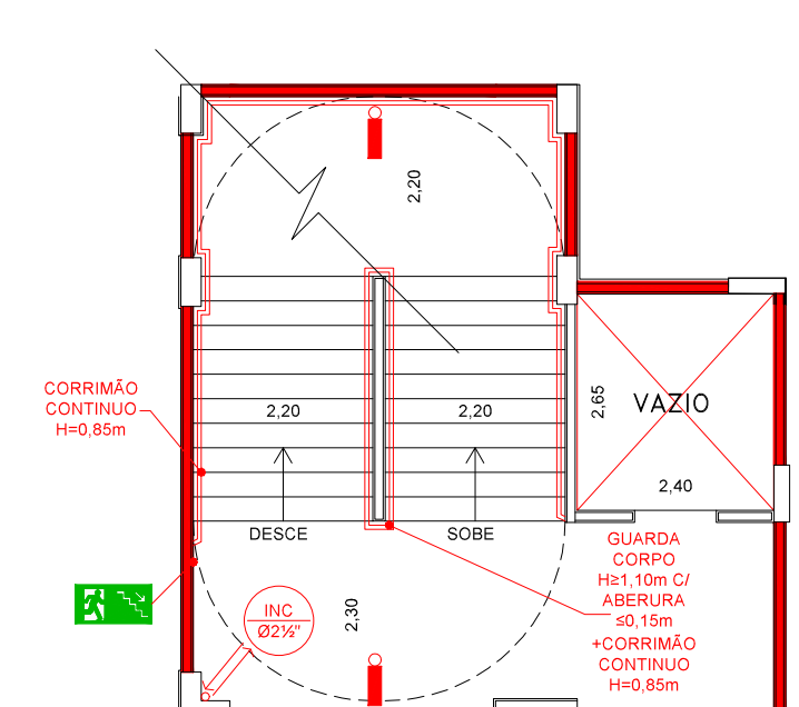
ESCADA INTERMEDIÁRIA (X5) SANTA CASA BLOCO A CASA DE MÁQUINAS ESCALA 1:100
