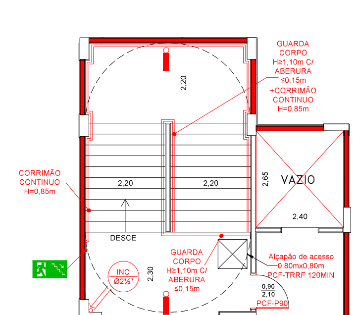
ESCADA INTERMEDIÁRIA (ACESSO AO BARRILETE) SANTA CASA BLOCO A CASA DE MÁQUINAS ESCALA 1:100
