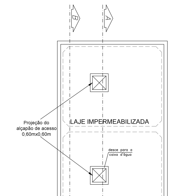
COBERTURA CAIXA D'ÁGUA SANTA CASA BLOCO A ESCALA 1:100
