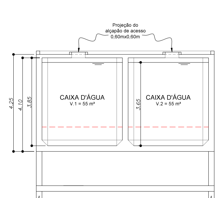
COBERTURA CAIXA D'ÁGUA SANTA CASA BLOCO A ESCALA 1:100
