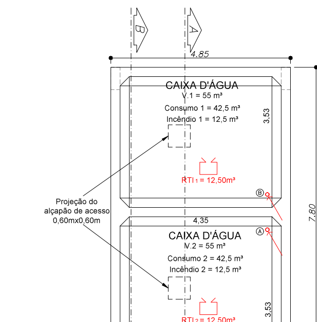
CAIXA D'ÁGUA SANTA CASA BLOCO A ESCALA 1:100
