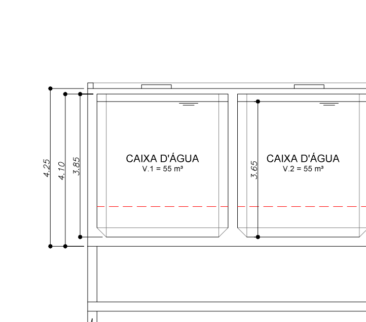
CORTE B-B CAIXA D'ÁGUA E BARRILETE ESCALA 1:100
