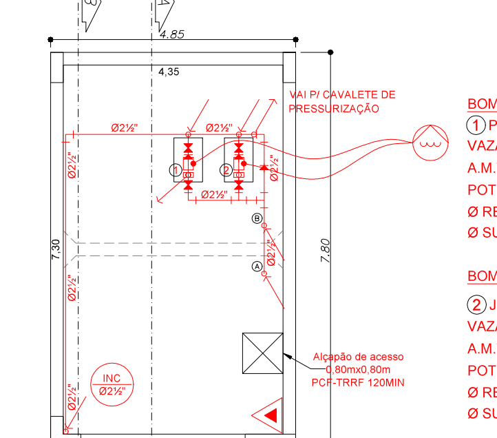
BARRILETE SANTA CASA BLOCO A ESCALA 1:100
