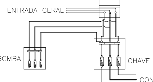
DETALHE LIGAÇÃO DA BOMBA SEM ESCALA
